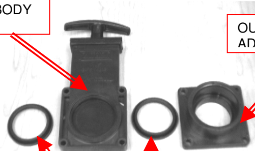
GASKET – NM3019
